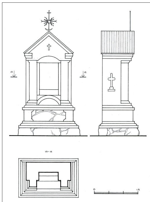
14 pav. Veprių šventoriaus koplytėlės planas (XXXIII Kryžiaus kelio stotis). Sudarė A. Rupeika. 2009 m.
