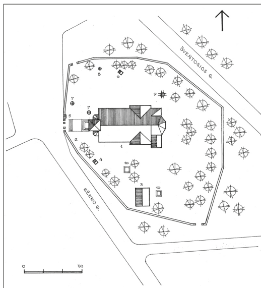
9 pav. Veprių bažnyčios statinių komplekso situacijos plano schema. Sudarė A. Rupeika. 2009 m.
