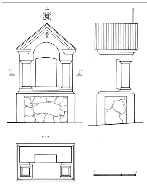
13 pav. Veprių šventoriaus koplytėlės planas (XXXV Kryžiaus kelio stotis). Sudarė A. Rupeika. 2009 m.
