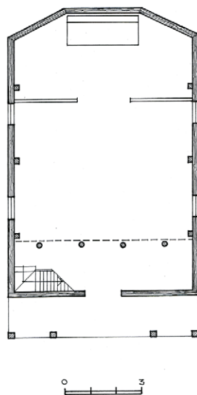
16 pav. Sližių kapinių koplyčios planas. Sudarė A. Rupeika. 2009 m.
