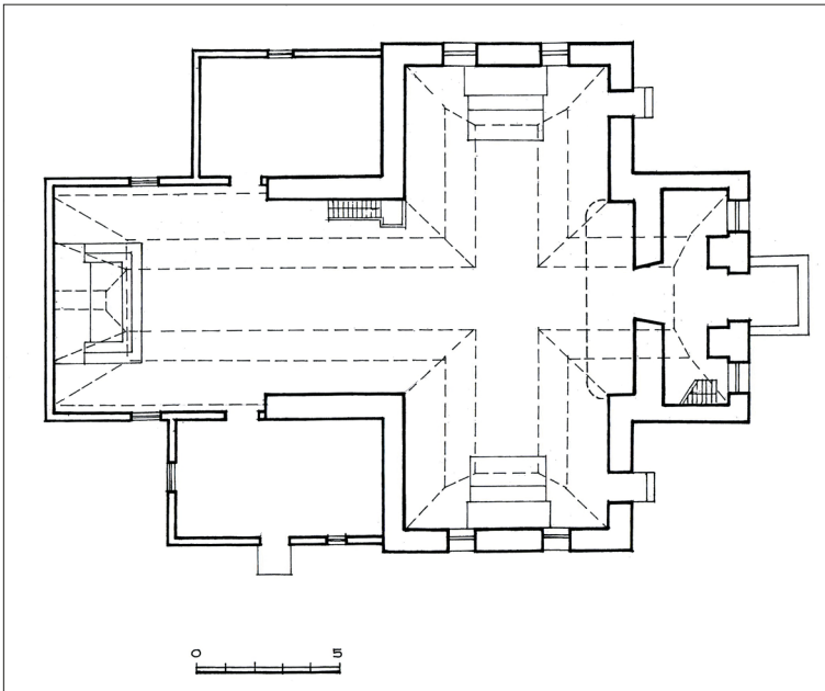
18 pav. Upninkų bažnyčios planas. Sudarė A. Rupeika. 2009 m.
