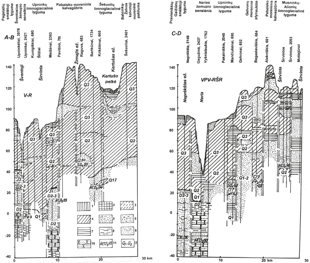
6 pav. Veprių apylinkės vidurinės dalies geologinis profilis. A–B (Upninkėliai–Šešuoliai).
