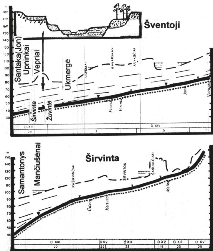
14 pav. Šventosios ir Širvintos upėkritis išilginiai profiliai. Mažasis slėnio profilis (aukštai) atspindi slėnio sandarą netoli Veprių (salpa ir 3 terasos). Žemėjančių linijų spektras – apytikriai terasų segmentai ir aukščiai
