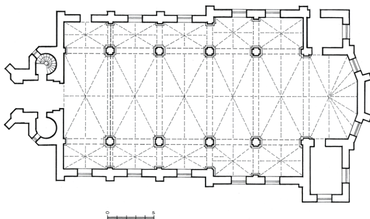
11 pav. Veprių bažnyčios planas. Sudarė A. Rupeika. 2009 m.
