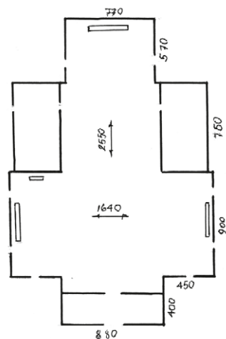
Upninkų bažnyčios schematinis planas. Sudarė autorius
