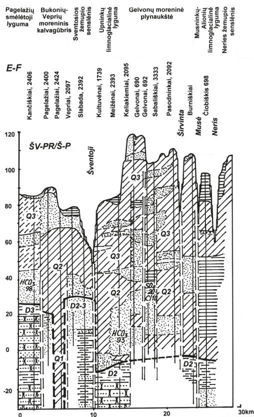
8 pav. Veprių apylinkės šiaurinės ir rytinės dalių geologinis profilis. E-F (Kančiškiai–Čiobiškis)
