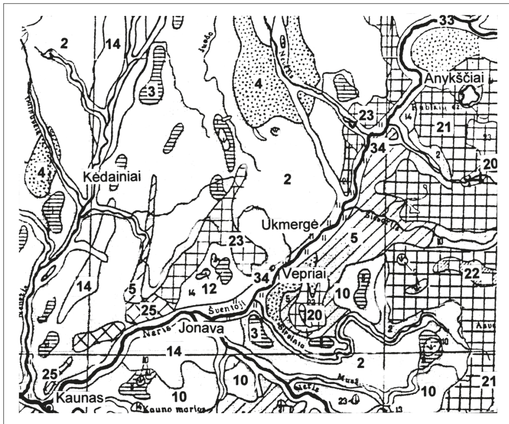
9 pav. Šventosios baseino ir Veprių apylinkės vietovaizdžių tipai pagal Žemėvaizdžius (A. Basalykas, 1981)
