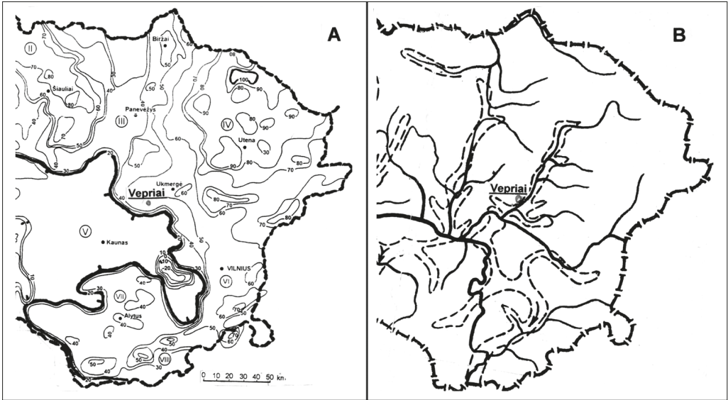
4 pav. A – Pokvarterinio (ledynų paliktos dangos pridengto) paviršiaus pavidalas. Ryškėja stambios reljefo pakopos bei lygumos. Tarp Jonavos ir Veprių glūdinti pakopa viršija 20 m (A. Šliaupa, 2000); B – po kvartero danga slypinčių upių slėnių, pažymėtų punktyrine linija, santykis su dabartiniu upynu (pagal V. Baltrūną, A. Šliaupą, 1980)
