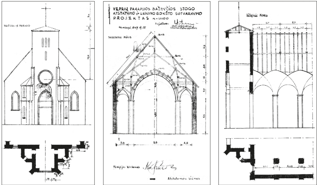
Veprių parapijos bažnyčios stogo atstatymo ir laikino bokšto sutvarkymo projektas: a) vaizdas iš priekio, b) skersinis pjūvis, c) išilginis pjūvis
