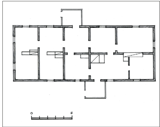
20 pav. Upninkų klebonijos planas. Sudarė A. Rupeika. 2009 m.
