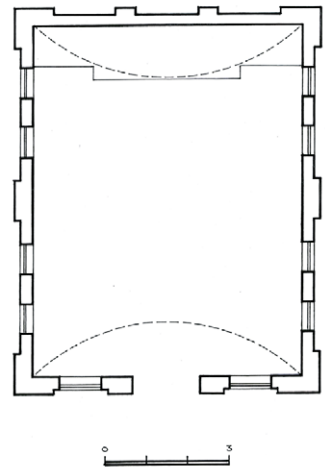
12 pav. Veprių šventoriaus koplyčios planas. Sudarė A. Rupeika. 2009 m.
